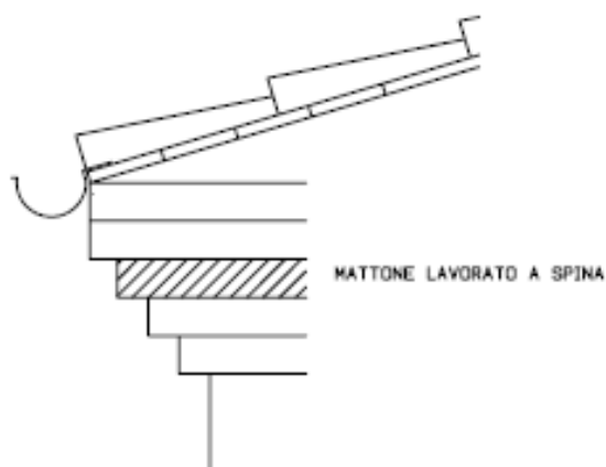
CORNICE IN MATTONI FACCIA VISTA
