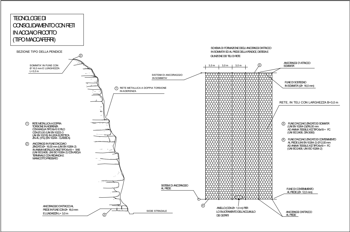
Schema delle reti di consolidamento superficiale
