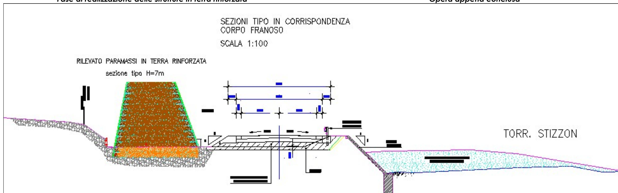
Fase di realizzazione delle strutture in terra rinforzata
