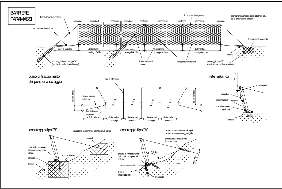
Schema della barriera paramassi
