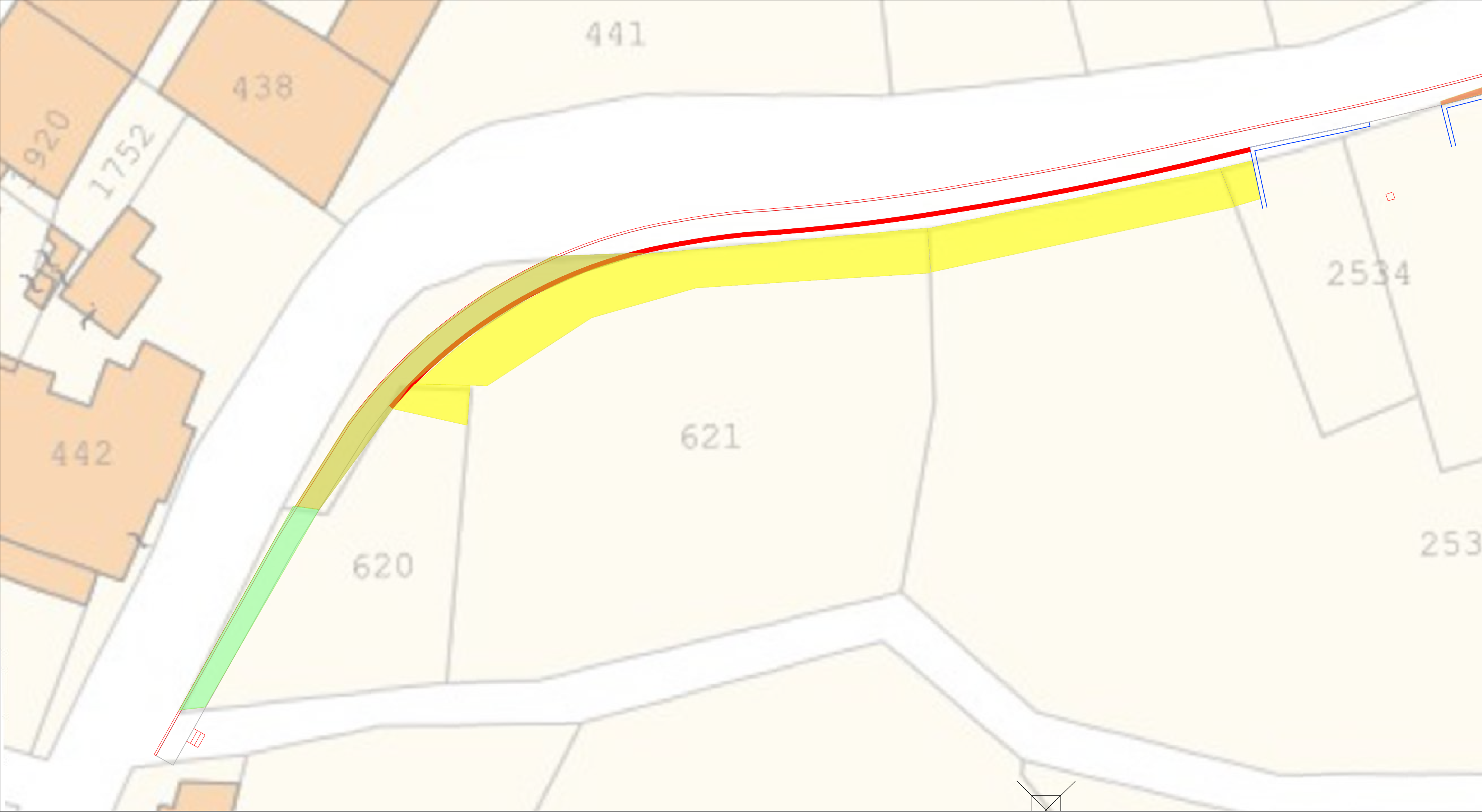
PLANIMETRIA CATASTALE CON INDIVIDUAZIONE ESPROPRI E OCCUPAZIONI - SCALA 1:200
