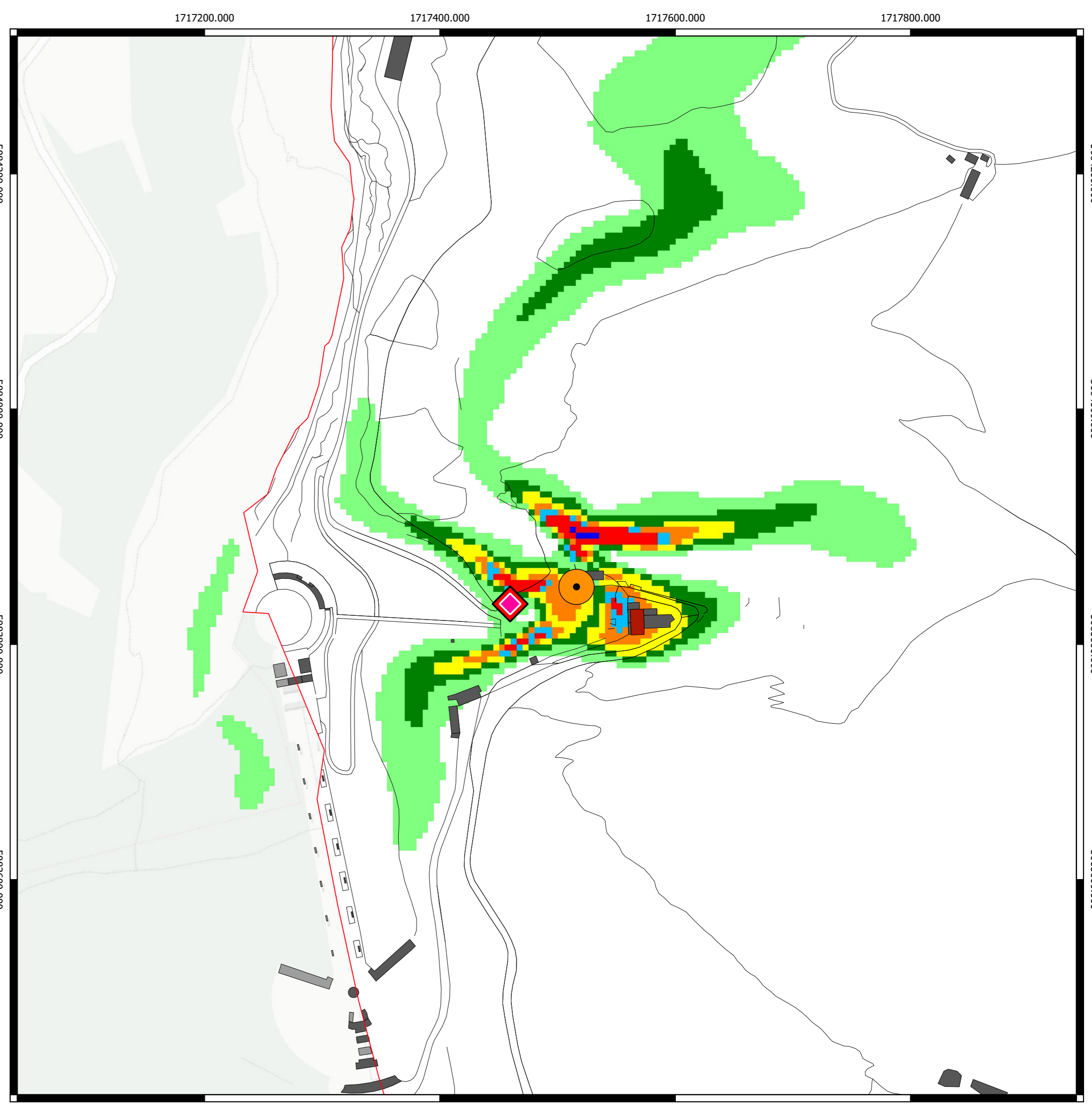
Campo elettromagnetico (V/m) calcolato alla quota di 9,38 m sul livello del terreno
