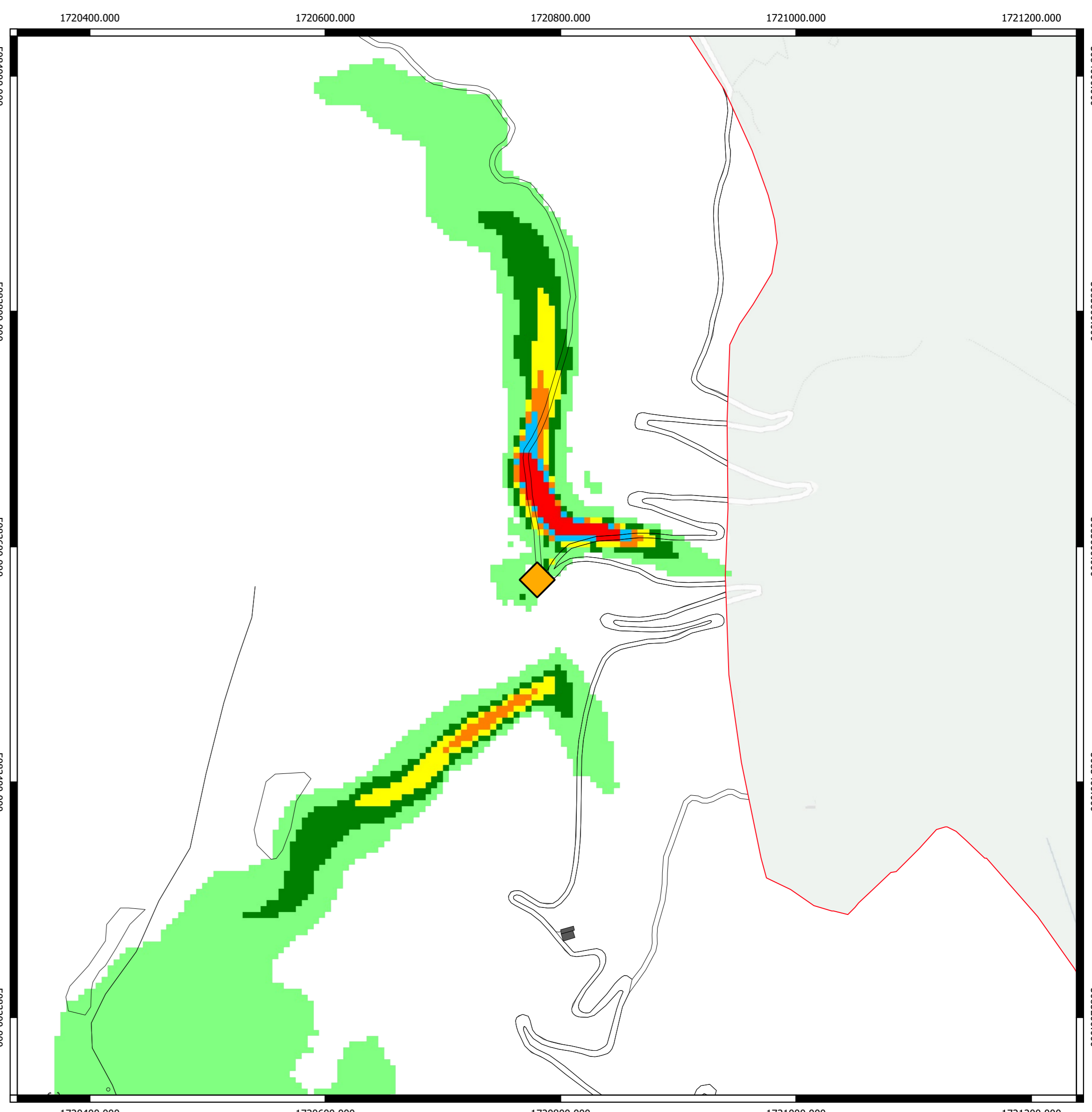
Campo elettromagnetico (V/m) calcolato alla quota di 5,66 m sul livello del terreno
