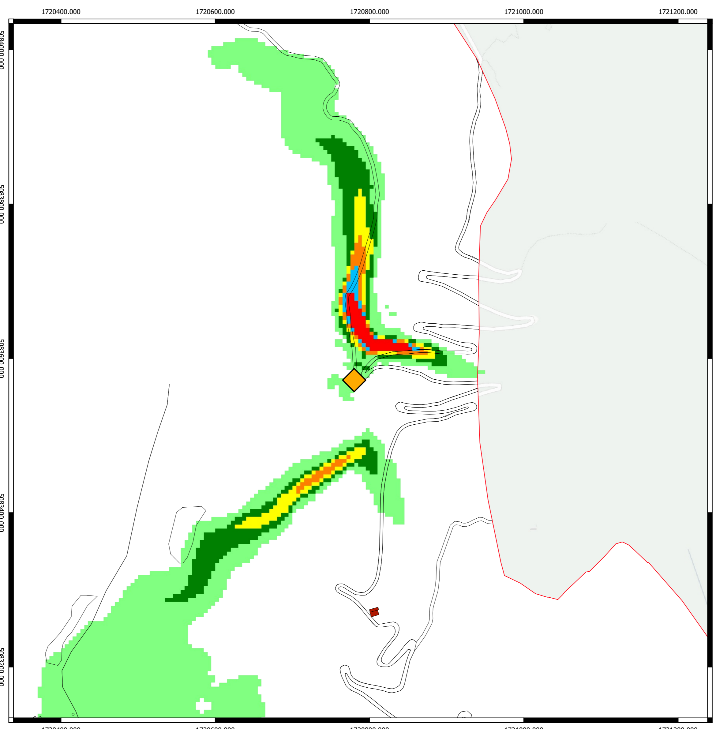
Campo elettromagnetico (V/m) calcolato alla quota di 3,66 m sul livello del terreno
